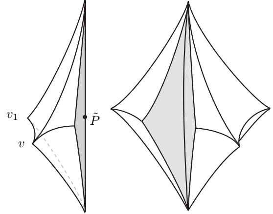
FIGURE 7. Découpage de \mathcal{T}
